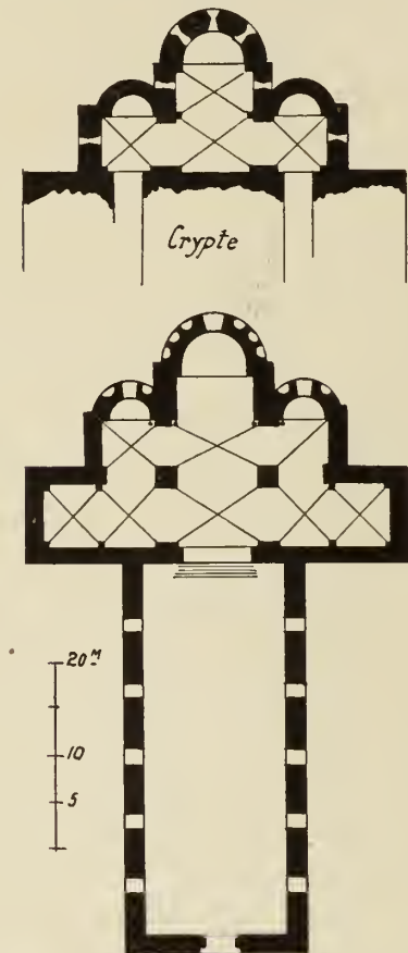
10630. — La Roccelletta. Plan de l'église et de la crypte. D'après Em. Bertaux, L'art dans l'Italie méridionale , 1904, t. I, p. 127, fig. 44.
